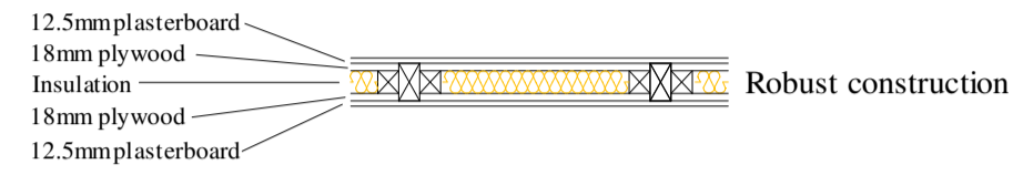
Stud partition
